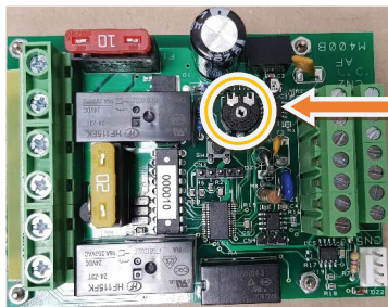
TRIMMER REGOLAZIONE VELOCITÀ
